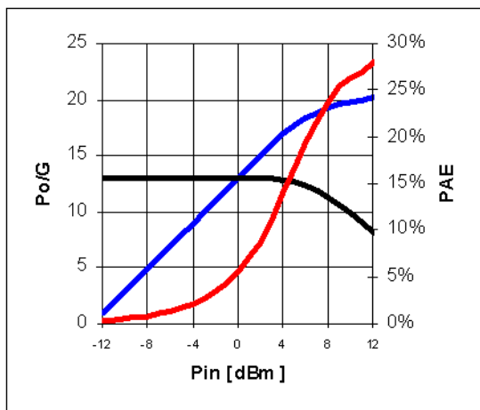
900MHz, 5V/70mA
